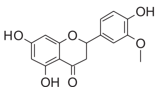
Hesperitin (2)
